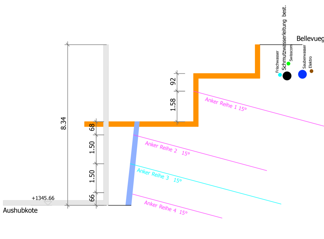
Schnitt Bellevuegässli QP 7
