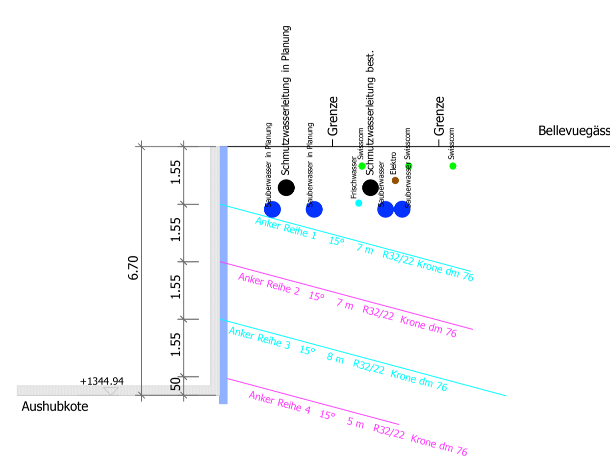
Schnitt Bellevuegässli QP 5
