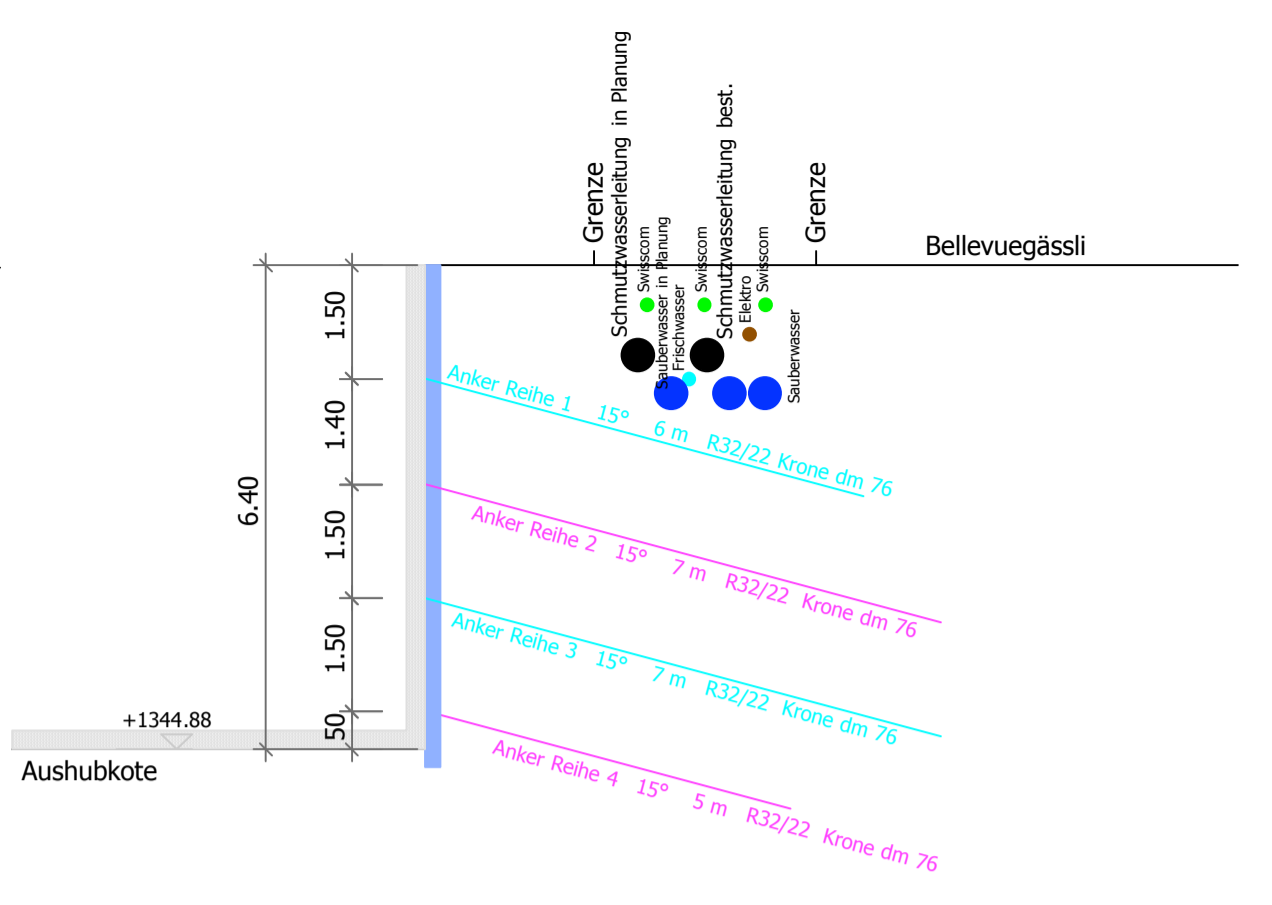
Schnitt Bellevuegässli QP 4
