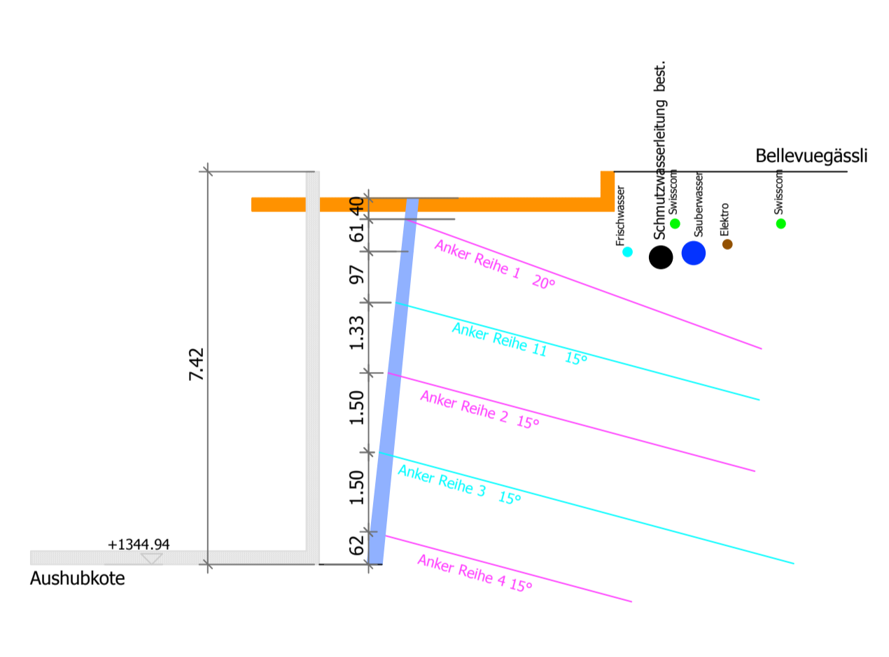
Schnitt Bellevuegässli QP 6
