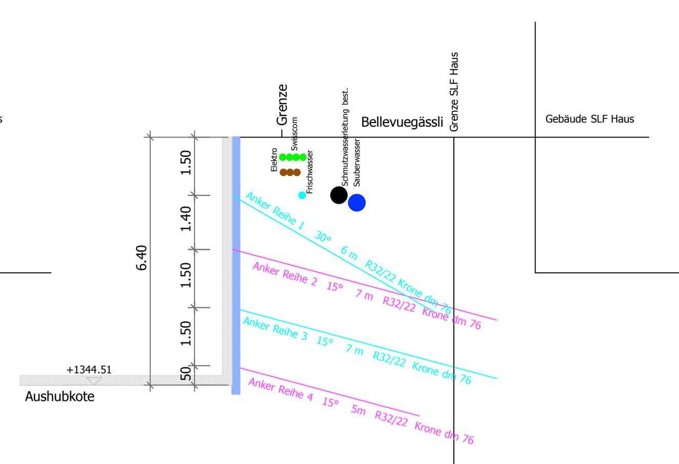
Schnitt Bellevuegässli QP 2
