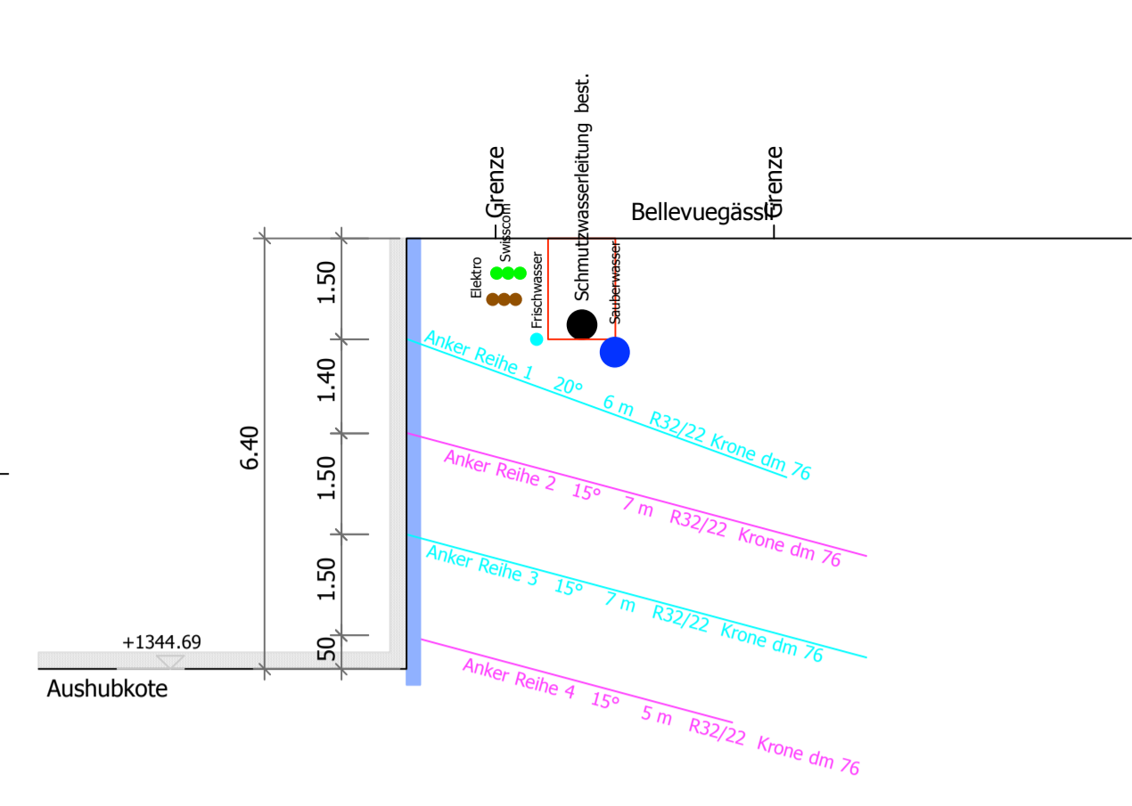
Schnitt Bellevuegässli QP 3
