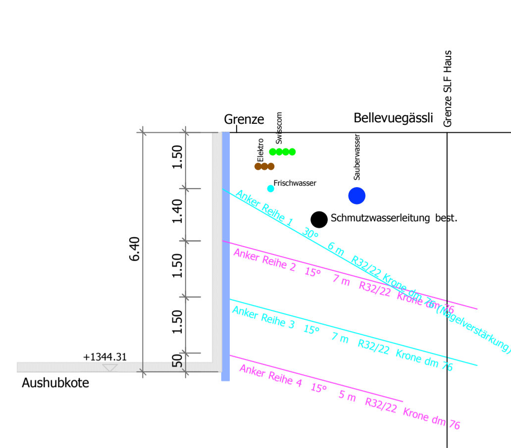
Schnitt Bellevuegässli QP 1
