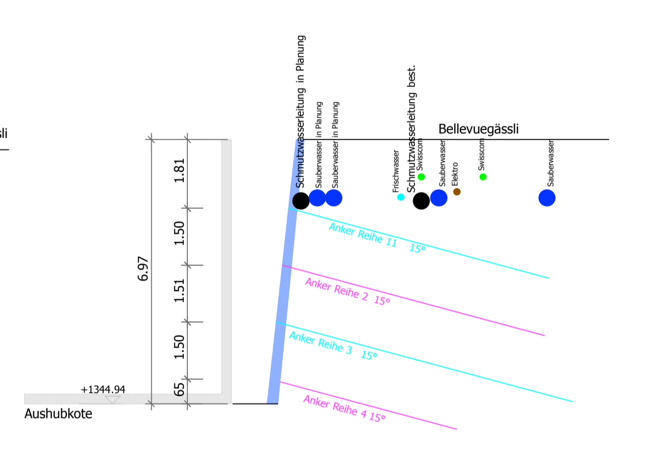
Schnitt Bellevuegässli QP 5.5
